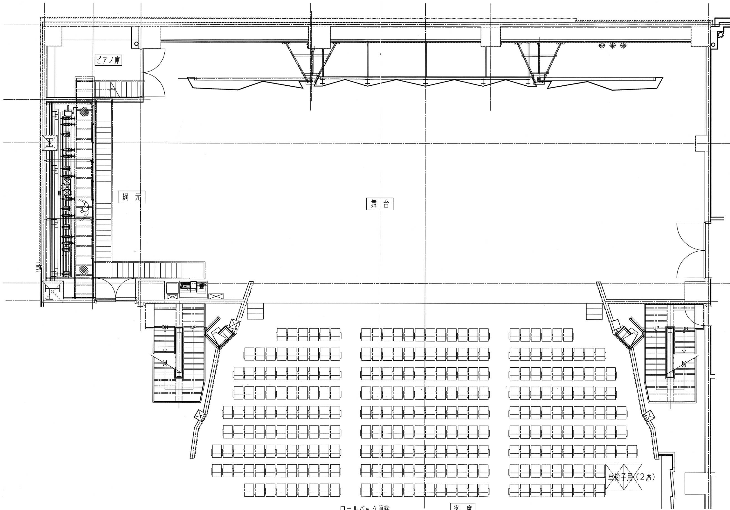
大ホール平面図 S=1/50
